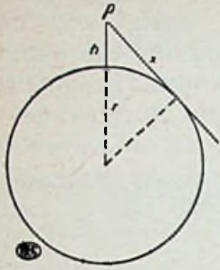
Fig. 1. Grootte der werkingssfeer x bij hoogte h van den zender.
