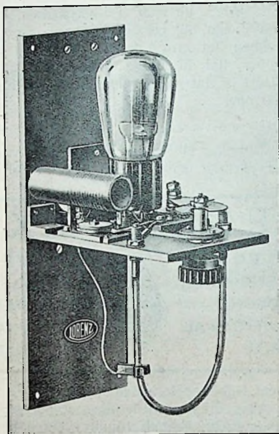
Fig. 3. Het hoogfrequent-gedeelte van den voor de proeven gebruikten 3-meter-zender.
