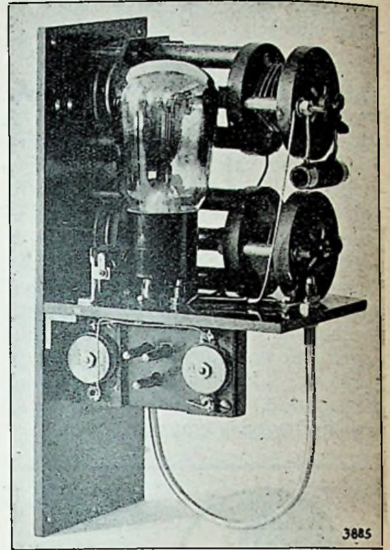
Fig. 4. Het hoogfrequent-gedeelte van den voor de proeven gebruikten 3-meter-ontvanger.
